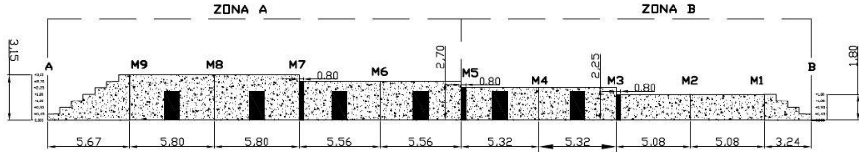
ALZADO FACHADA
